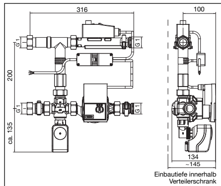
Abb. 4.1 Abmessungen
