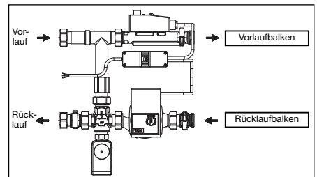
Abb. 6.2 Durchflussrichtung
