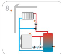
Circuit de chauffage mélangé avec chaudière à combustible
