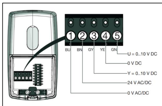
PIN-Zuordnung
