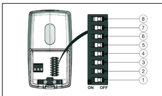
DIP-Schalter
