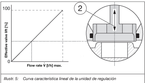
Illustr. 5: Curva característica lineal de la unidad de regulación
