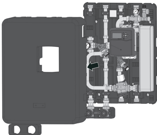
Abb. 26: Wärmedämmoberschalen entfernen
