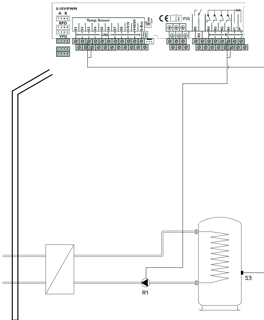
Abb. 51: Schema 7, indirekte Trinkwassererwärmung
