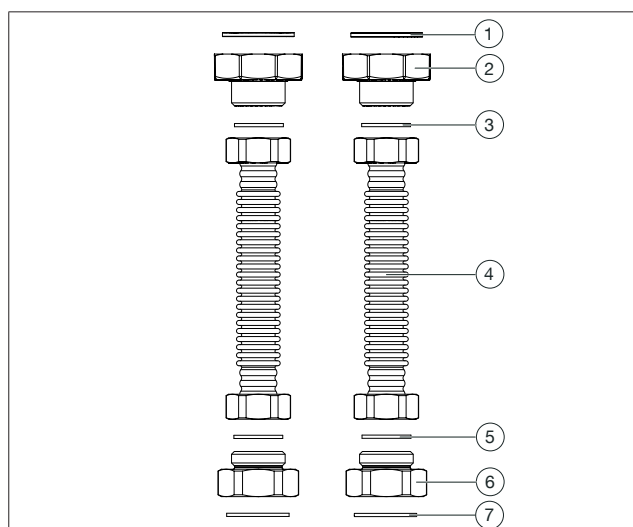
Abb. 29: Aufbau Verbindungsset
