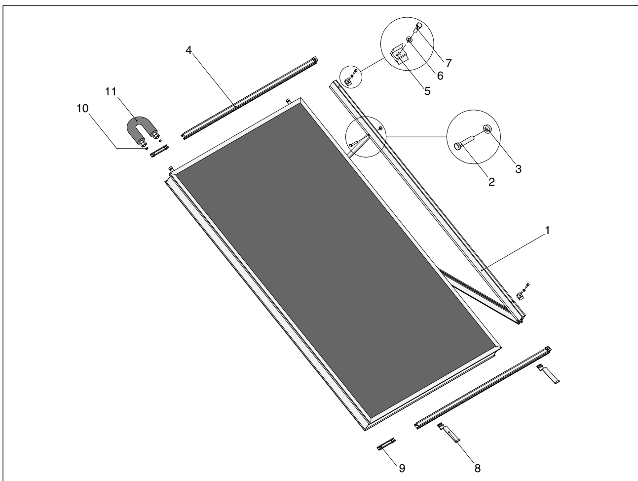
Erweiterungsset Freiaufstellung Art.-Nr. 136 12 87 (Kollektoren nicht im Lieferumfang enthalten)
