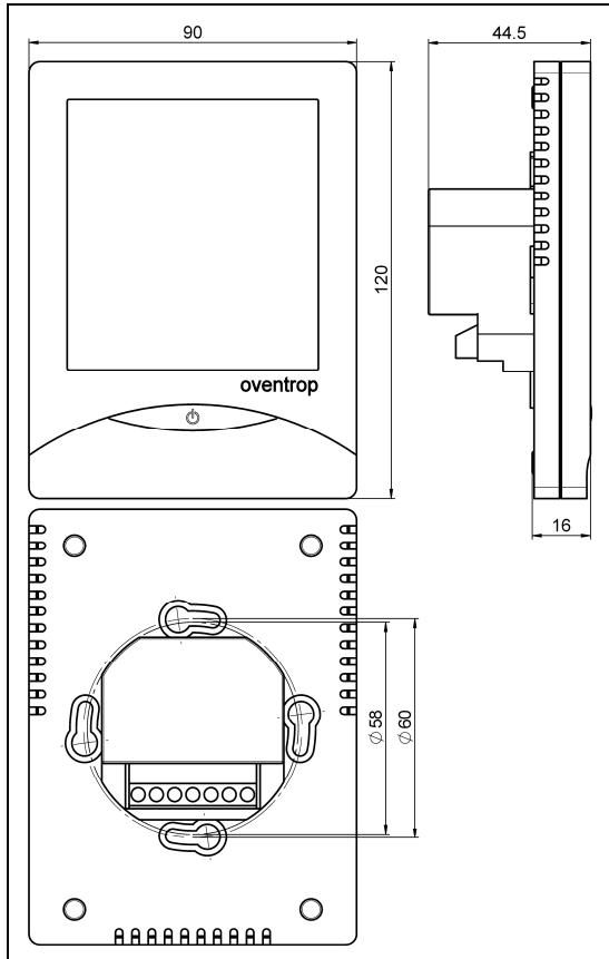
Abb. 4.1 Abmessungen
