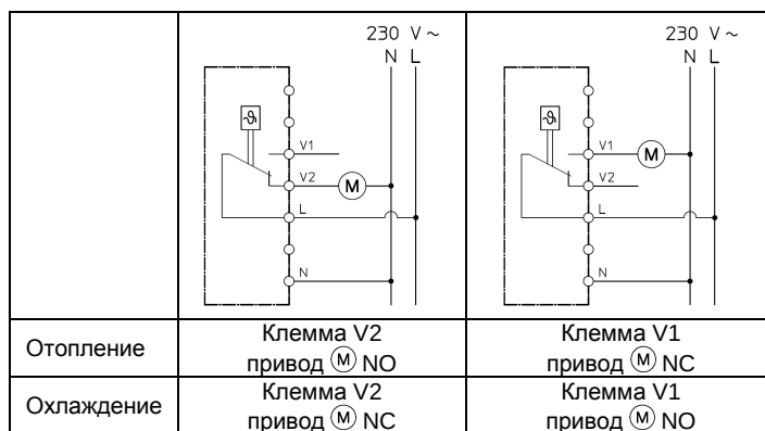
Рис. 6.1 Схема подключения отопление/охлаждение
