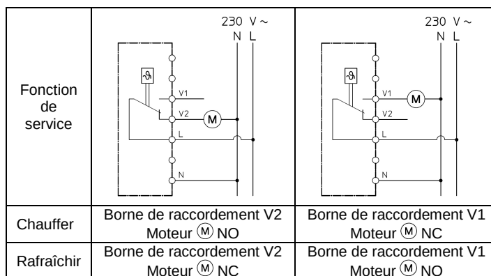
Fig. 6.1 Schéma électrique Chauffer/rafrâchir
