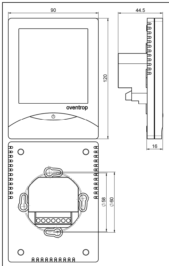
Fig. 4.1 Encombres
