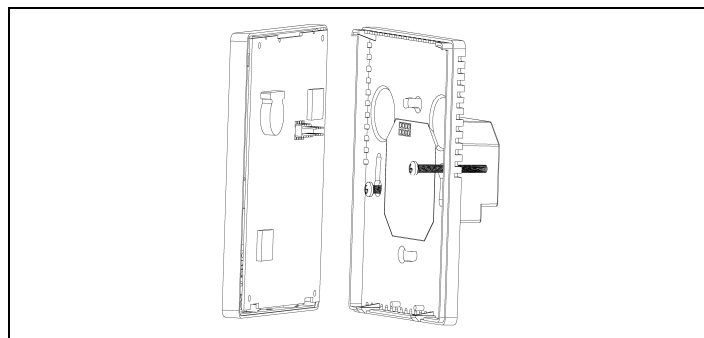
Fig. 6.2 Montage du thermostat
