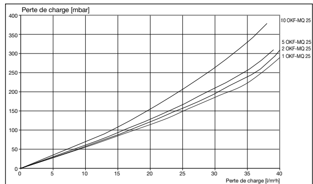
Fig. 7: Perte de charge pour plusieurs capteurs interconnectés en fonction du débit; fluide caloporteur: 40% glycol / 60% eau à 40°C; perte de charge incluant tuyaux de raccordement
