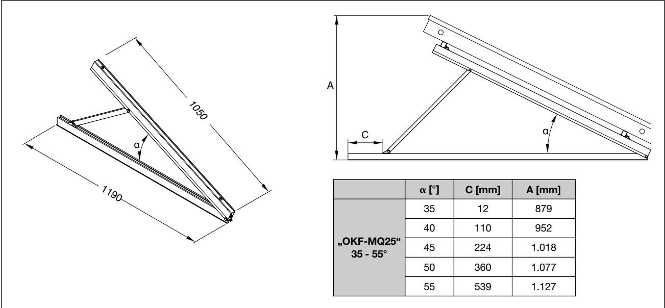
Abb. 22: mögliche Aufstellwinkel
