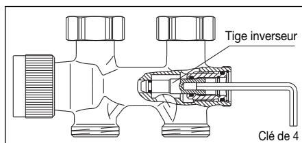
Fig. 8 Transformation en service monotube
