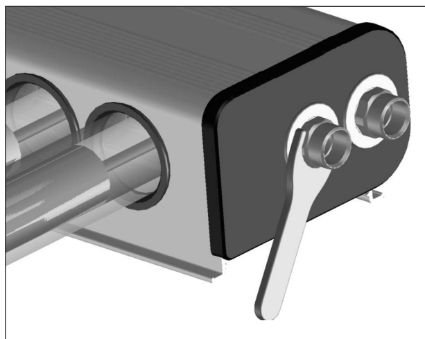
Abb. 29: Kollektoranschlüsse gegenhalten
