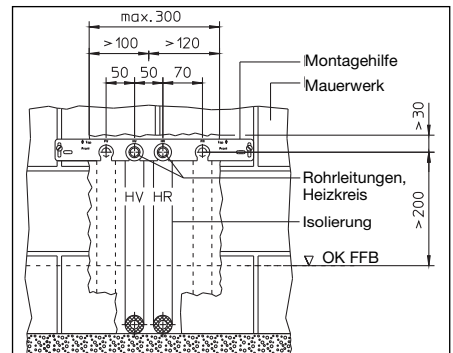
Abb. 7 Wandansicht, Heizkreisanschluss
