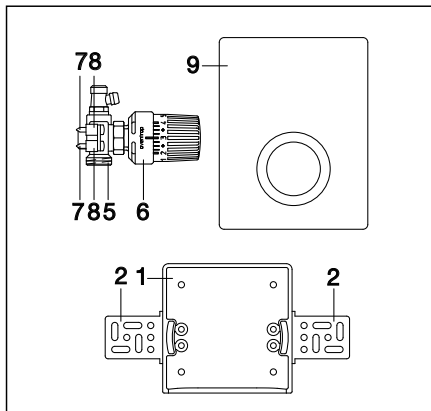
Samenstelling ombouwset
