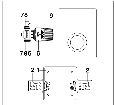
Komponenten Umrüstsatz
