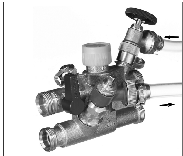
Bild/Illustr./Fig. 7 Spülen des abgesperrten Sekundärkreises Flushing of isolated terminal Rinçage du circuit secondaire fermé
