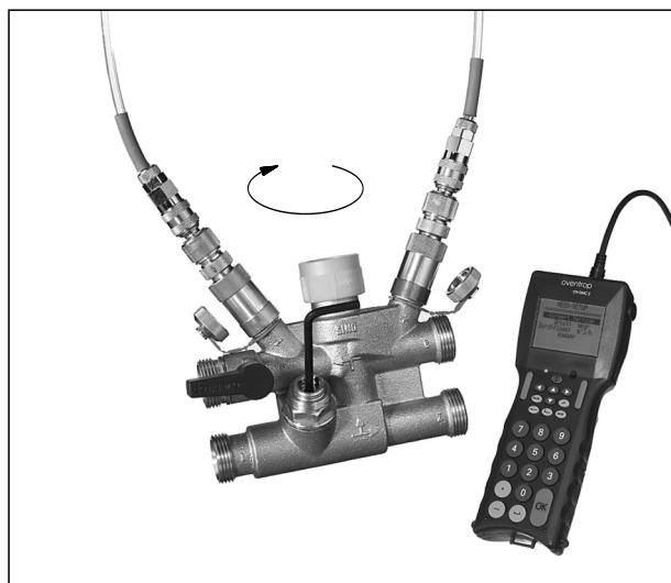
Bild 2/Illustr./Fig. 2 Voreinstellen mittels Differenzdruckmessung Presetting by differential pressure measurement Préréglage moyennant la mesure de la pression différentielle
