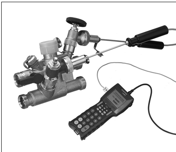
Bild/Illustr./Fig. 5 Messung der Temperatur des Sekundärkreises Temperature measurement of terminal unit Mesure de la température du circuit secondaire
