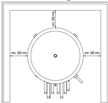
Fig. 3 Encombrenents de montage
