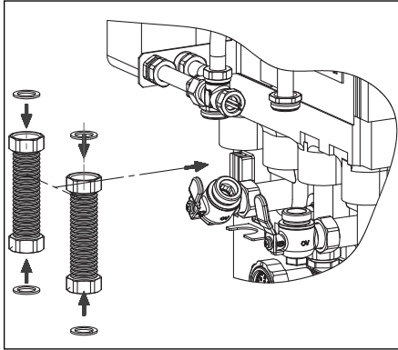
Abb. 14 Montage Metallwellrohre
