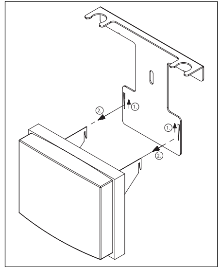
Abb. 16 Demontage Blinddeckel mit Halteblech
