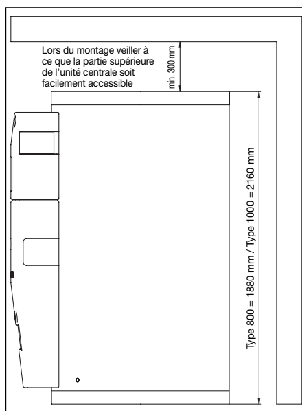
Fig. 4 Encombrenents de montage
