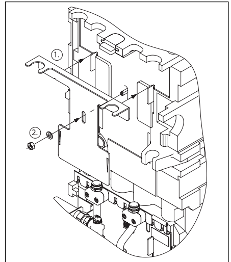
Abb. 17 Montage Solargruppenvorbereitung
