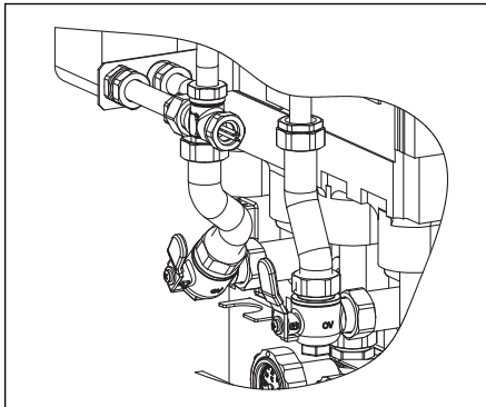
Abb. 15 Montage Metallwellrohre
