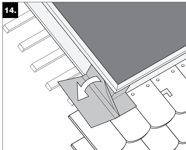
14. Hochstehenden Blechschenkel auf Eindeckung bündig andrücken.
