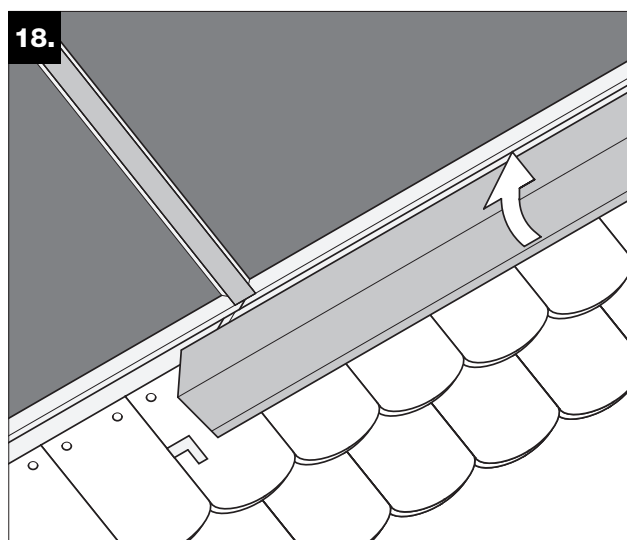
18. Untere Eindeckbleche einsetzen.
