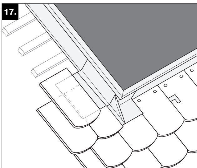
17. Jedes Blech passend mit einem Ziegel überdecken.
