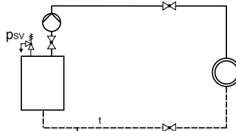
reflex 'V Vorschaltgefäß' nur für t \geq 70 \text{ }^\circ\text{C} reflex 'V In-line vessel' only for t \geq 70 \text{ }^\circ\text{C} in Heizungsanlagen In heating system
