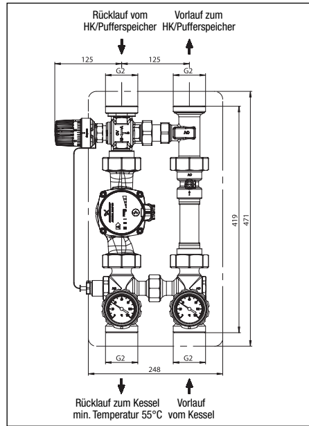
Abb. 4.6 „Regumat RTA-180“ DN32 mit Standardisierung Vorlauf auf der rechten Seite Kessel ist unterhalb der Station angeordnet
