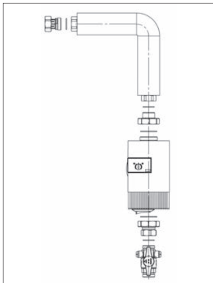
Fig. 1.5 Set di collegamento ricircolo con pompa Wilo Stratos PARA Z 25/1-12 RK e adattatori
