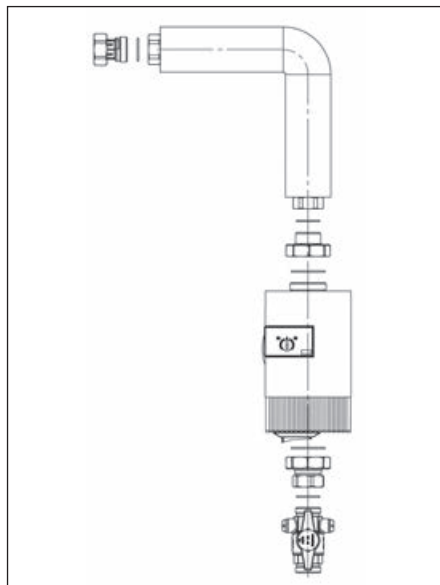
Abb. 1.5 Zirkulationsanschluss- Set mit Pumpe Wilo Stratos PARA Z 25/1-12 RK und Adaptern
