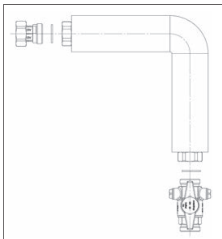
Abb. 1.3 Zirkulationsanschluss- Set Trinkwasser- Zirkulationspumpe bauseits montiert
