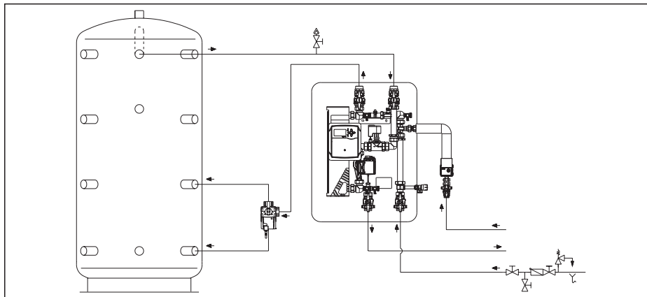
Fig. 1.6 Esempio di installazione
