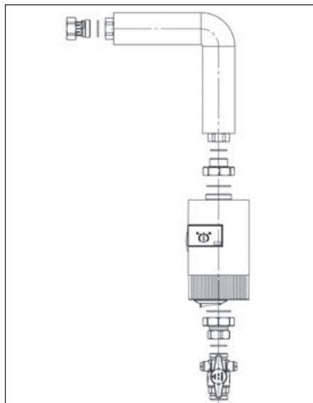
Fig. 1.5 Jeu de raccordement de bouclage avec circulateur Wilo Stratos PARA Z 25/1-12 RK et adaptateurs
