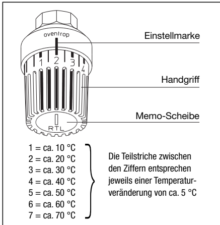
Abb. 3 Temperaturvorhalte-Regelset
