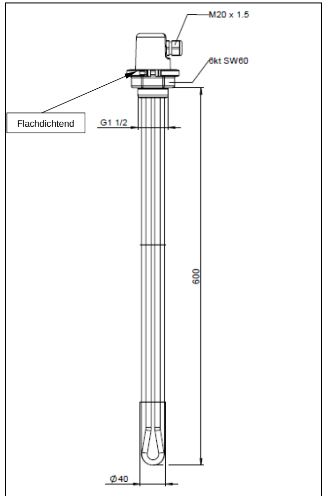
Abb. 4.1 Abmessungen
