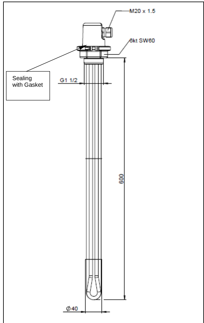
Fig. 4.1 Dimensions
