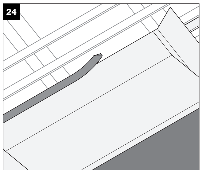
24. Schwarzes Schaumgummiband auf das obere Abdeckblech entlang des Falzes kleben.
