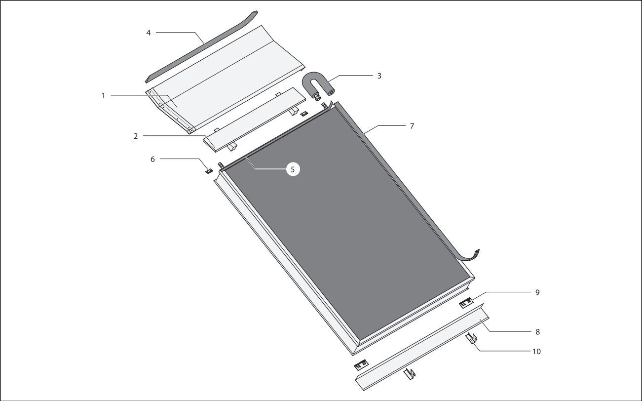
Set d'extension pour intégration en toiture, réf. 136 12 94 (les capteurs ne sont pas fournis avec)
