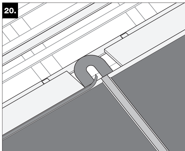
20. Coller le ruban d'étanchéité en caoutchouc cellulaire sur le cadre supérieur du capteur.
