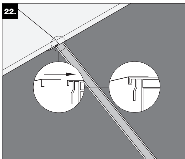
22. Placer la tôle de raccordement en haut et la faire coulisser dans la rainure du collecteur avec la rainure en tôle.
