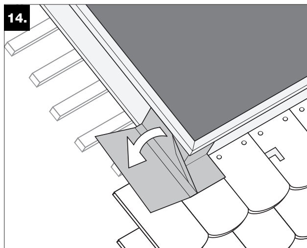
14. Presser à fleur la partie verticale de la tôle sur la couverture.
