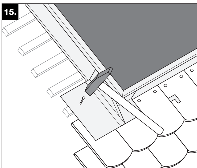
Die einzelnen Seitenbleche mit Dachpappennägeln auf Dachlatten befestigen.
