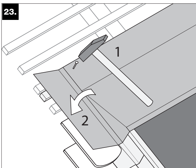
23. Clouer les tôles de raccordement sur les lattes et ajuster la partie verticale de la tôle aux coins comme décrit ci-dessus.
