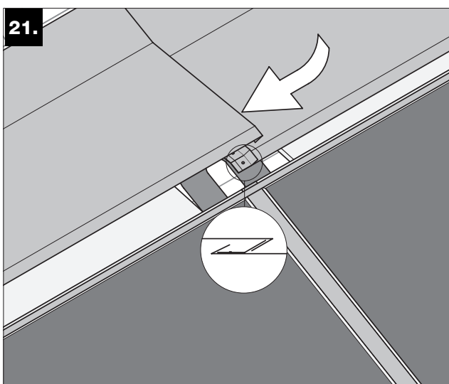
21. Accrocher les tôles de raccordement en haut aux rainures intérieures l'une après l'autre et les fixer entre elles à l'aide du collier au verso.
