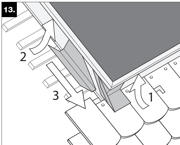
Die beiden Teile des Eckstücks in die tiefere Kollektornut einsetzen (1 + 2) und zusammenschieben (3).
