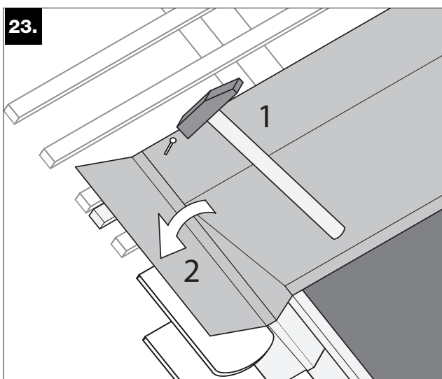
23. Obere Abschlussbleche auf Latten nageln und an den Ecken den hochstehenden Blebschenkel anpassen wie zuvor beschrieben.
