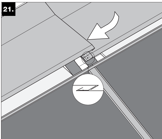
21. Obere Anschlussbleche nacheinander an den inneren Falzungen ineinanderhaken und mit der rückseitigen Lasche untereinander fixieren.
