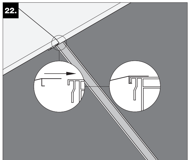
22. Oberes Abschlussblech auflegen und mit Blechnut in Kollektorfalz einschieben.
