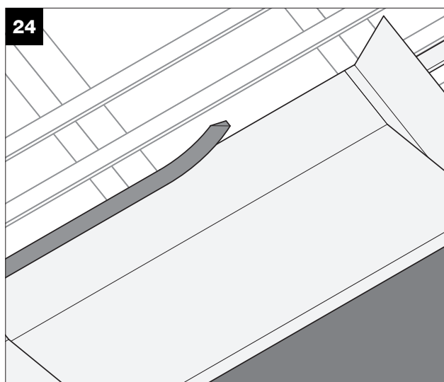
24. Coller le ruban d'étanchéité noir en caoutchouc mousse sur la tôle de protection en haut le long de la rainure.
