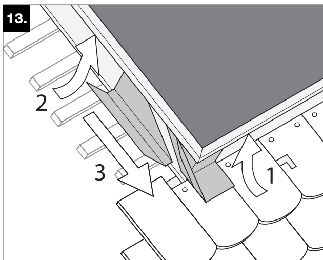
13. Introduire les deux parties du gousset dans la rainure inférieure du capteur (1 + 2) et les rapprocher (3).
