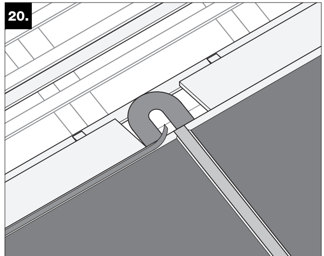
20. Zellgummidichtband auf oberen Kollektorrand aufkleben.
