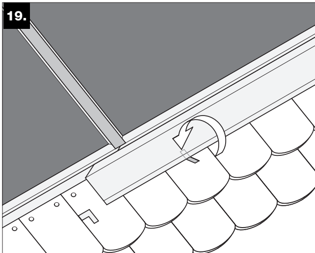
19. Untere Eindeckbleche mit Blechklammern fixieren.
