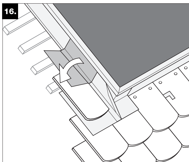
16. Introduire les tôles dans la rainure inférieure, les aligner au bord supérieur de la latte du haut et les monter à recouvrement sur chaque rangée de tuiles avoisinante en partant du bas vers le haut.
