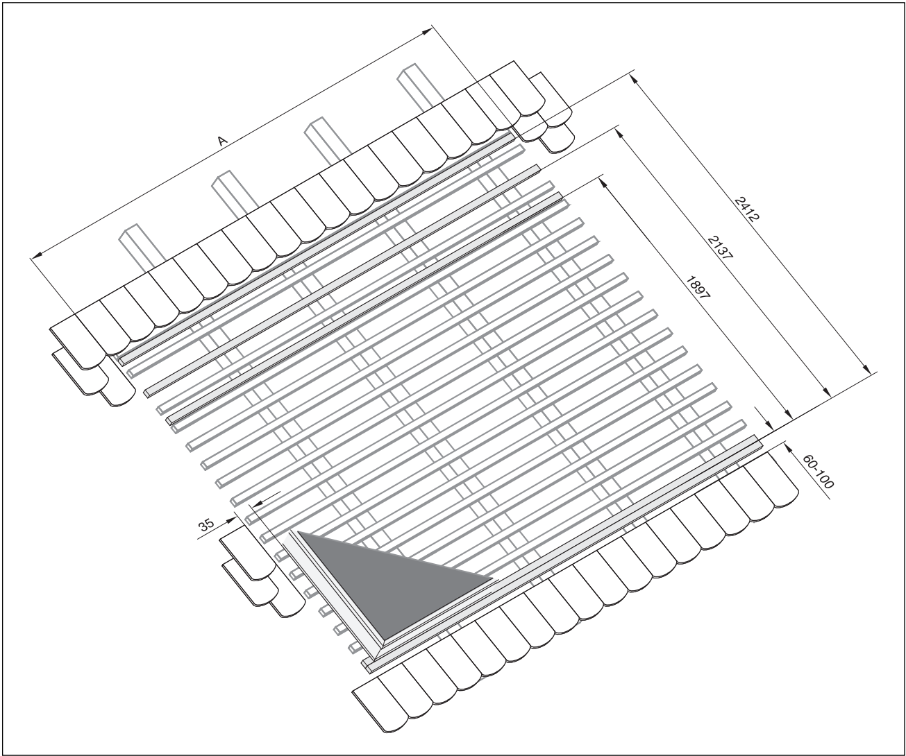
Cotes de la zone de montage et positionnement des lattes de montage. Epaisseur des lattes à choisir selon les lattes de toit existantes. Les lattes de toit nécessaires en sus sont marquées de couleur grise (5 pièces) ; Longueur des lattes = A (largeur zone de montage) Dimensions extérieures du capteur (L x l) = 1930 x 1160
