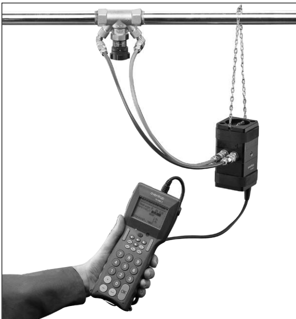
Durchflussmesscomputer Art.-Nr. 1069177
