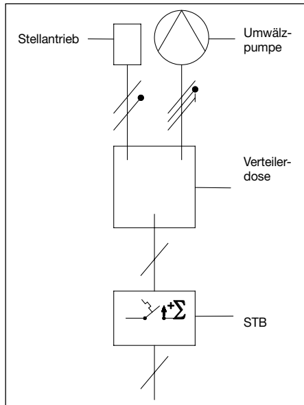
Abb. 4.1 Systemdarstellung Verkabelung
