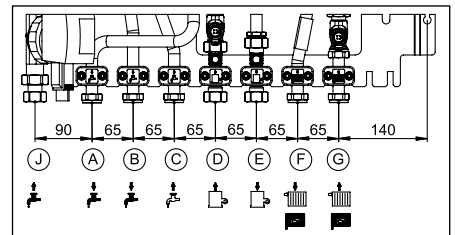
Fig. 4.4 Cotes de raccordement
