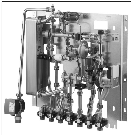
Abb. 1.1 „Regudis W-HTF“ Wohnungsstation mit Zirkulationsleitung
