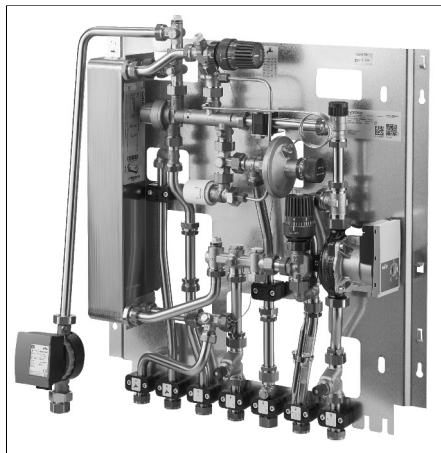
Fig. 1.1 Modulo satellite “Regudis W-HTF” con ricircolo
