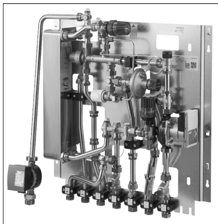
Fig. 1.1 Station d'appartement «Regudis W-HTF» avec conduite de bouclage d'E.C.S.
