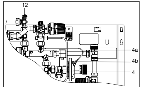
Illustr. 8.2 Bleeding
