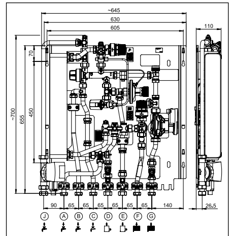
Fig. 4.3 Encombrements avec circuit de chauffage mélangé et conduite de bouclage d'E.C.S.
