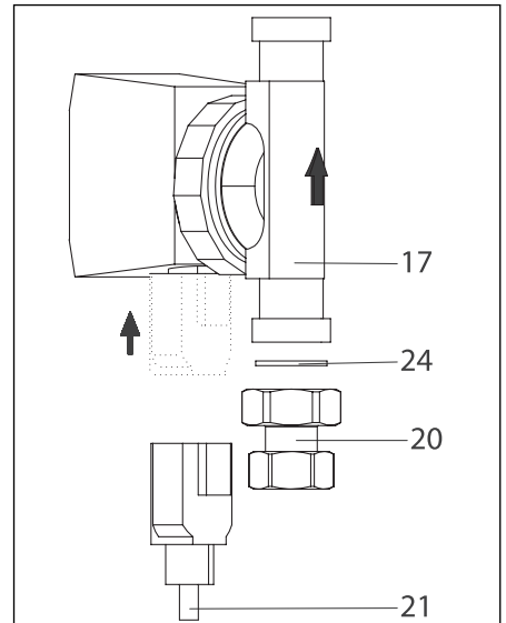
Fig. 6.2 Orientation du circulateur
