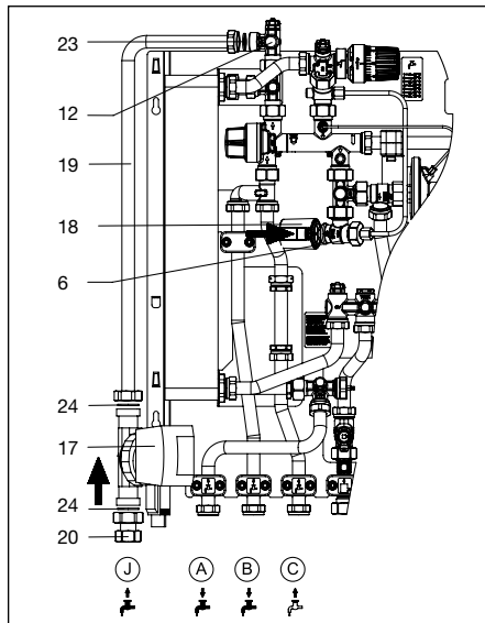
Fig. 6.1 Montaggio
