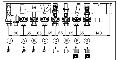
Abb. 4.4 Anschlussmaße
