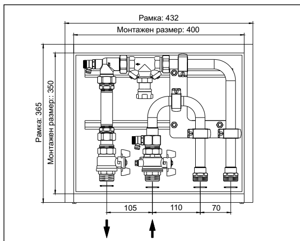
Размери на „Floorbox UV“, вертикално свързване на щранга
