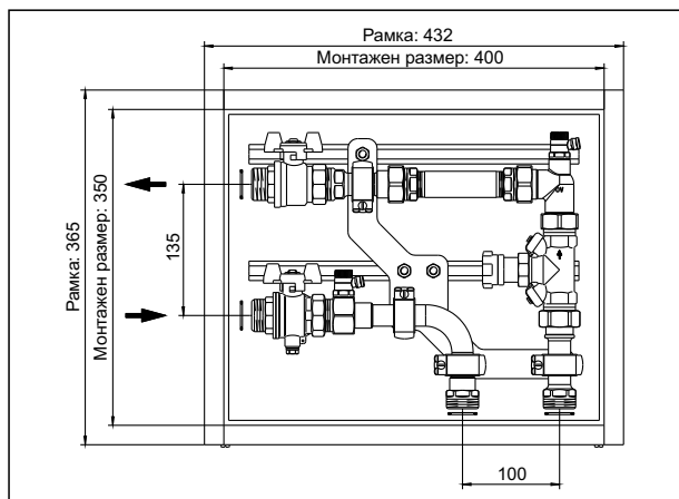
Размери на „Floorbox UH“, хоризонтално свързване на щранга
