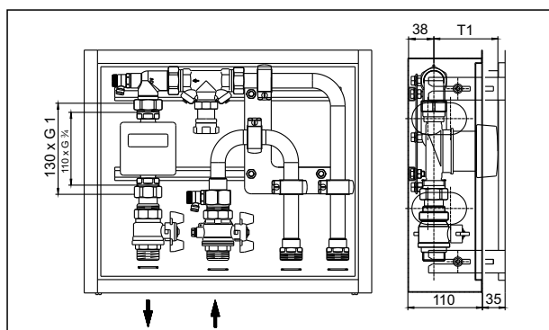
Монтажна дълбочина на „Floorbox U“
