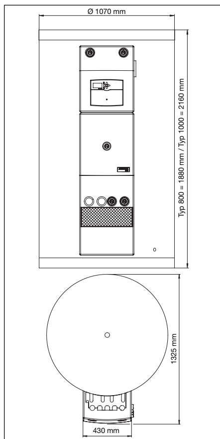
Fig. 2 Dimensioni
