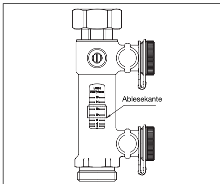
Abb. 36 Abgleichventil
