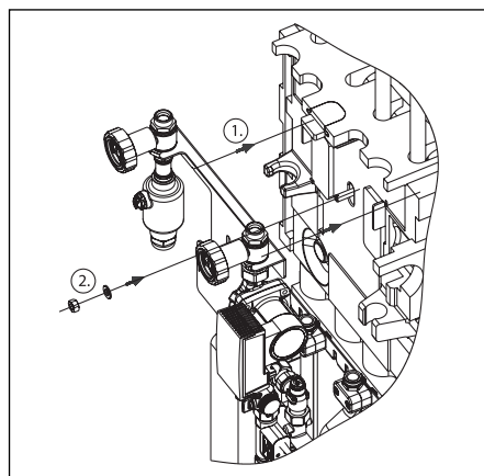
Fig. 17 Montage du groupe solaire
