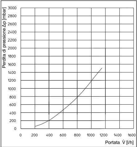
Perdita di pressione circuito secondario (acqua sanitaria) per funzionamento a ricircolo
