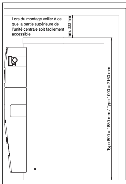
Fig. 4 Encombrements de montage
