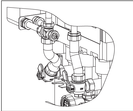
Abb. 15 Montage Metallwellrohre
