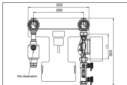
Fig. 37 Dimensioni "Regusol L 130 DN20"
