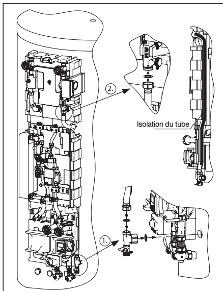
Fig. 20 Montage du tube annelé métallique retour solaire
