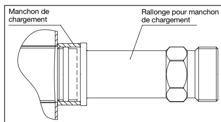
Fig. 5 Rallonge monté pour manchon de chargement
