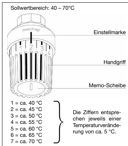
Abb. 34 Temperaturregler
