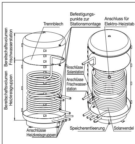
Abb. 43 Funktionsschnitt
