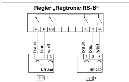
Abb. 27 Regler
