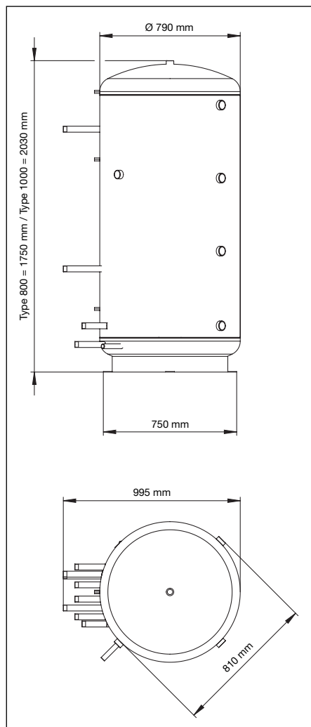
Fig. 42 Encombrements ballon d'eau chaude sans isolation
