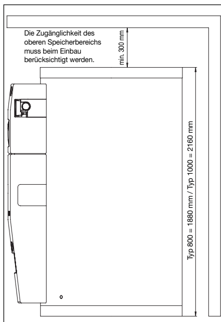
Abb. 4 Einbaumaße
