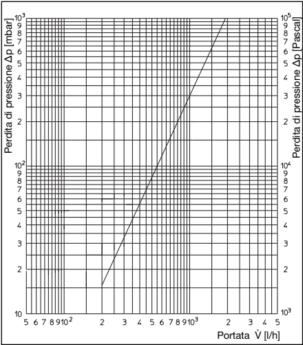
Perdita di pressione circuito primario (Circuito serbatoio) a massimo prelievo acqua calda sanitaria
