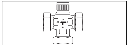
Abb. 50 Drei-Wege-Ventil für Zwei-Zonen-Beladung (1131706).
