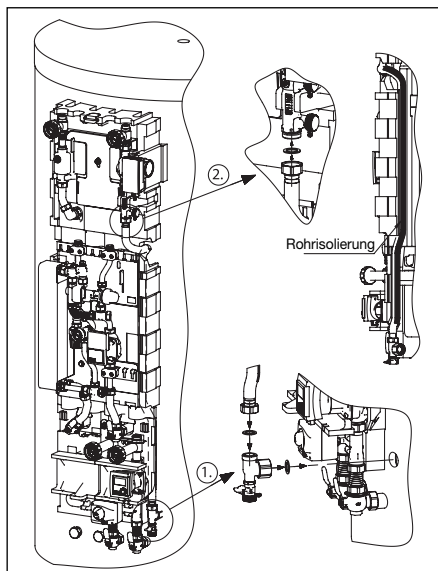
Abb. 20 Montage Metallwellrohr Solarrücklauf
