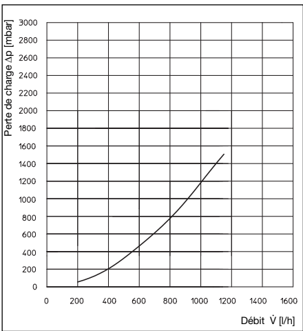
Perte de charge circuit secondaire (circuit eau potable) en service bouclage
