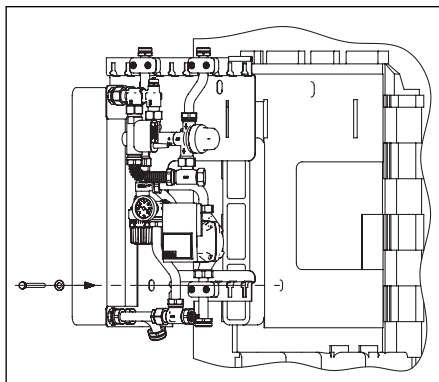
Fig. 12 Montaggio gruppo ACS
