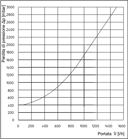
Perdita di pressione circuito primario (Circuito serbatoio) a massimo prelievo acqua calda sanitaria
