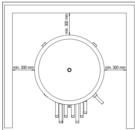
Abb. 3 Einbaumaße
