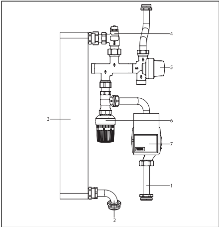
Abb. 31 Primärkreislauf
