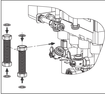
Abb. 14 Montage Metallwellrohre
