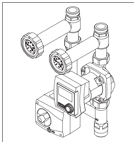
Abb. 25 „Regumat M3-130 DN20“
