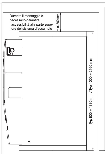
Fig. 4 Quote di montaggio
