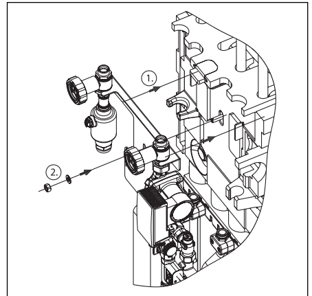
Abb. 17 Montage Solargruppe
