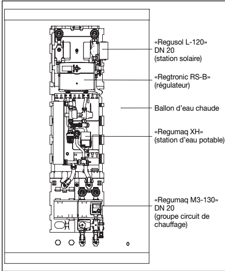
Fig. 24 Vue d'ensemble des composants
