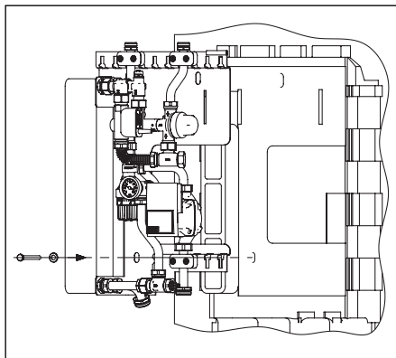
Abb. 12 Montage Frischwasserstation
