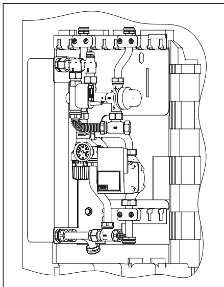
Abb. 13 Montage Frischwasserstation
