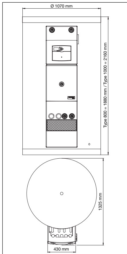
Fig. 2 Encombrements
