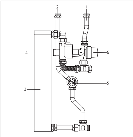
Abb. 32 Sekundärkreislauf
