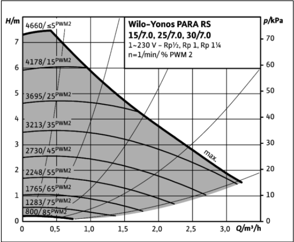
Courbe de fonctionnement Wilo-Yonos PARA RS 15/7
