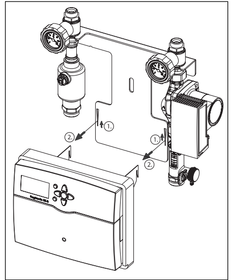
Abb. 16 Demontage Regler
