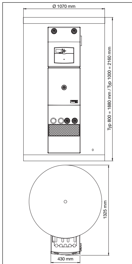
Abb. 2 Abmessungen
