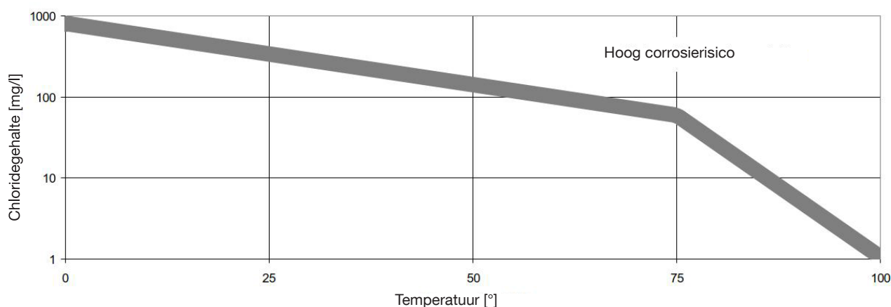
Toegestaan chloridegehalte afhankelijk van de temperatuur
