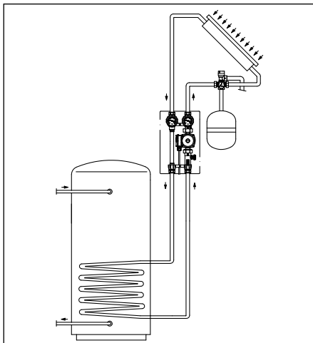
Ausdehnungsgefäß anschließen
