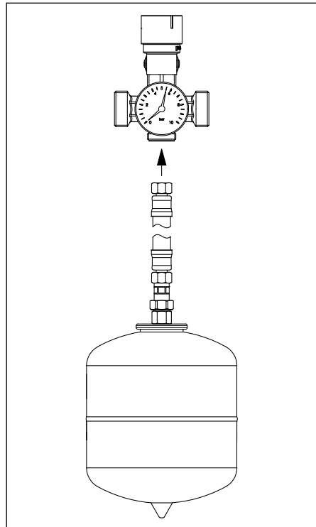
Ausdehnungsgefäß anschließen
