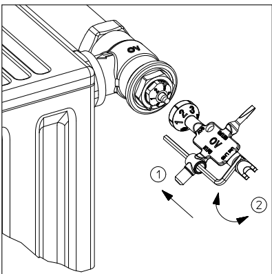
Voreinstellung Ventile „Baureihe AV6” / Ventileinsätze „GH” Presetting valves “Series AV6” / Valve inserts “GH” Préréglage robinets «Série AV6» / Mécanismes «GH»
