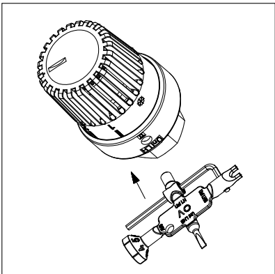
Demontage Handgriff Thermostat „Uni LH” Removal handgrip thermostat “Uni LH” Démontage poignée manuelle thermostat «Uni LH»
