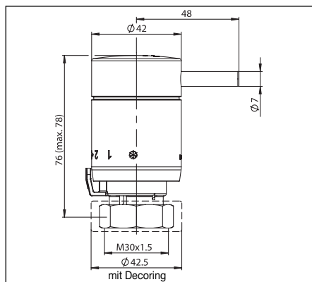
Abb. 4.1 Abmessungen
