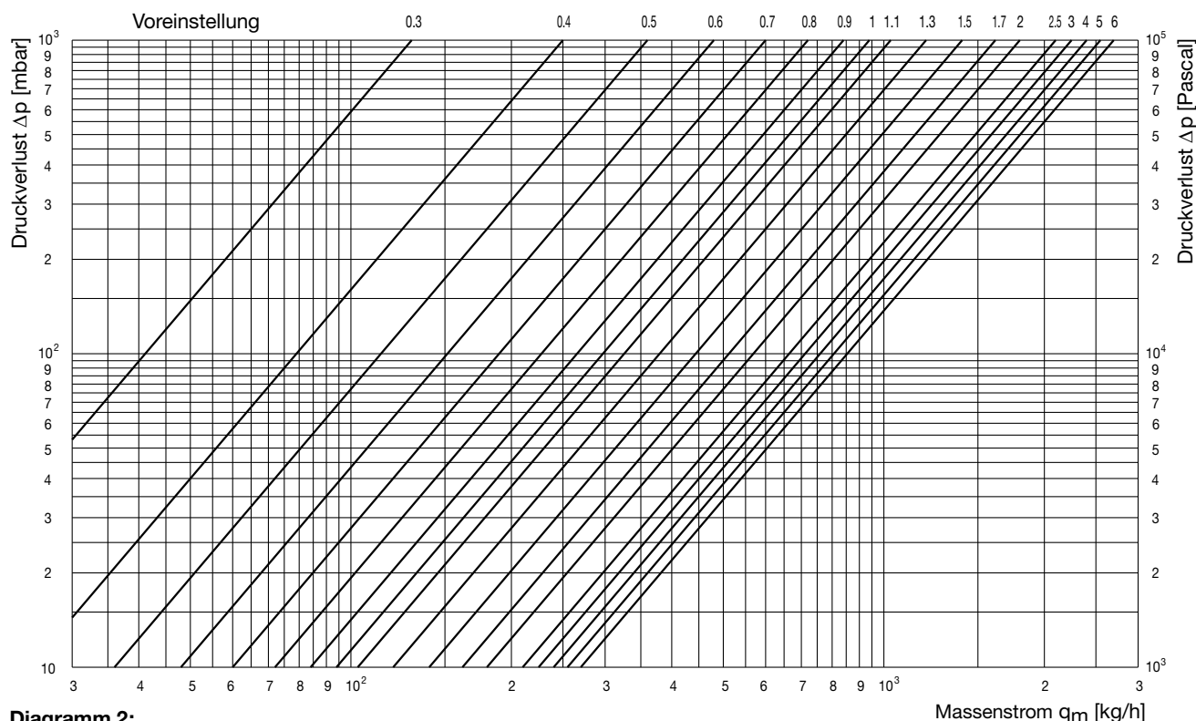
Diagramm 2: Druckverlust „Hycocn VTZ“ Strangreguliertventil DN 20
