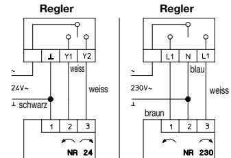
Dreipunktsteuerung
