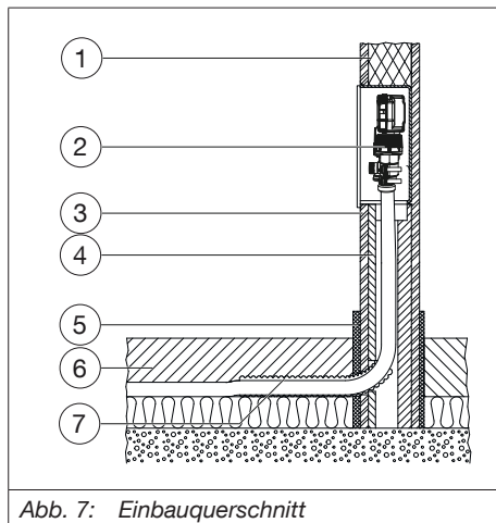
Abb. 7: Einbauquerschnitt
