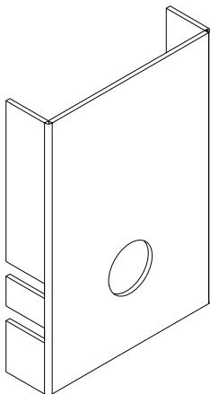
Fig. 1 : Capot de protection sur l'« Unibox T-RTL R-Tronic »
