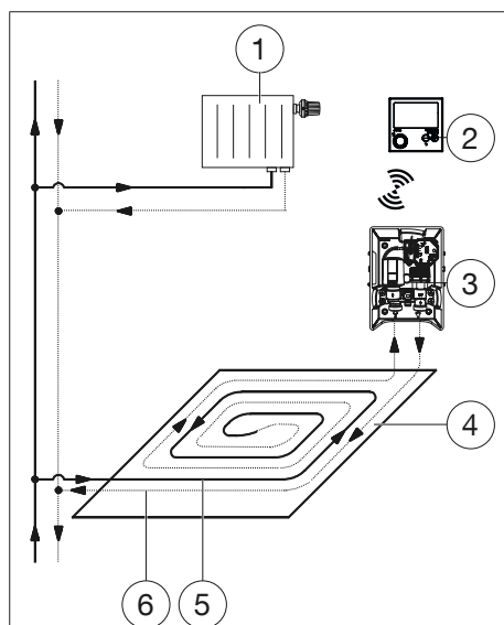
Fig. 8 : Raccordement
