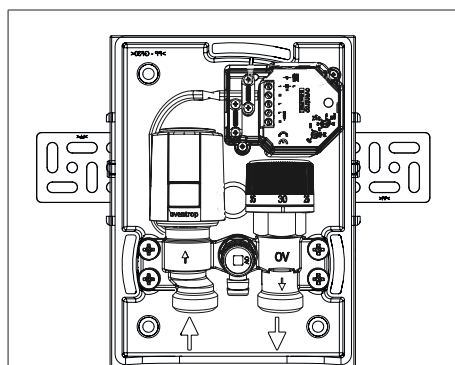
Fig. 9 : « Unibox T-RTL R-Tronic » avec équerres
