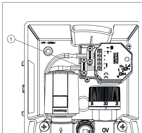
Abb. 10: Funkempfänger „R-CON FBH“ elektrisch anschließen
