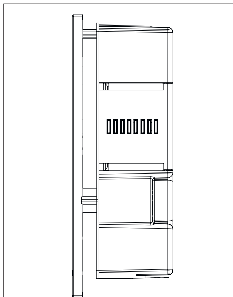
Fig. 6 : Capot extrait
