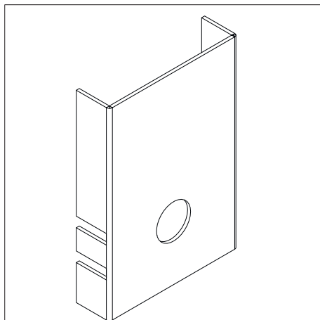
Abb. 1: Bauabdeckung auf „Unibox T-RTL R-Tronic“
