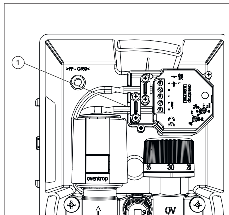
Fig. 10 : Branchement électrique du récepteur radio « R-Con FBH »
