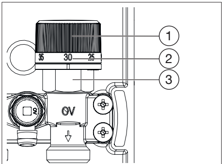
Fig. 4 : Poignée manuelle
