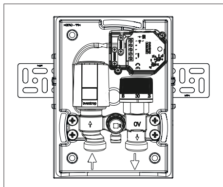
Abb. 9: „Unibox T-RTL R-Tronic“ mit Winkeln
