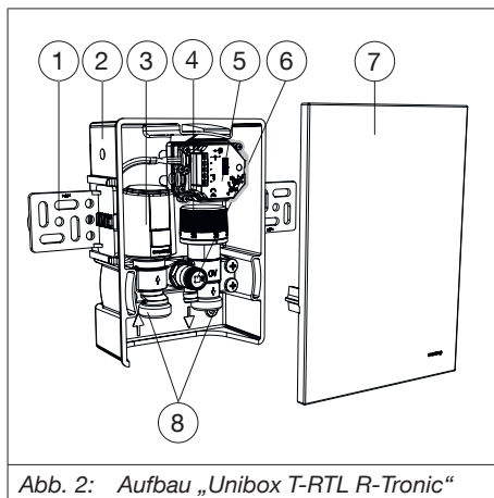
Abb. 2: Aufbau „Unibox T-RTL R-Tronic“
