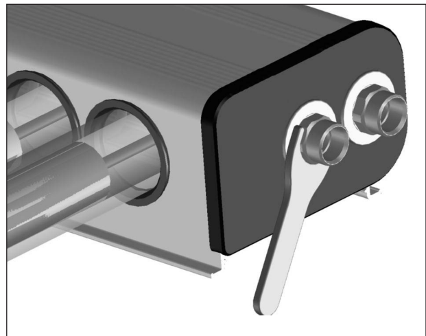
Abb. 29: Kollektoran- und -abflüsse gegenhalten
