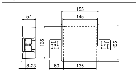
Encombrements
