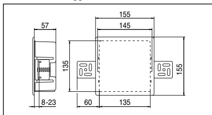
Dimensioni
