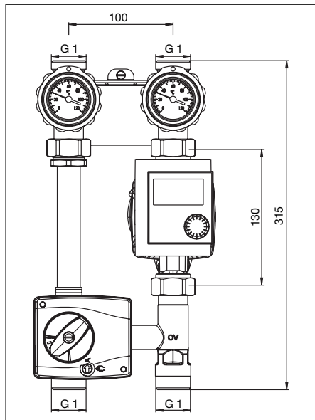
Fig. 4.1 Dimensions
