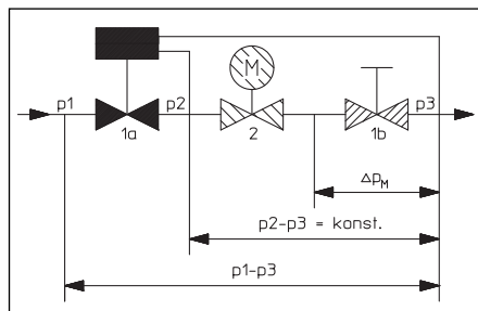
Abb. 5.3 Funktionsprinzip „Cocon QTZ“
