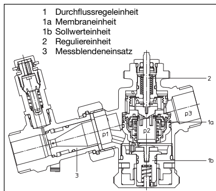
Abb. 5.2 Aufbau „Cocon QTZ“ mit Messblende
