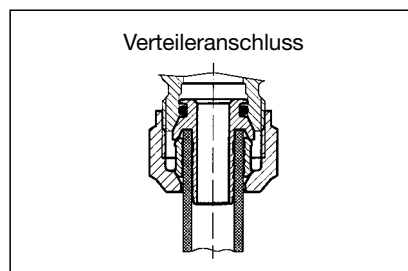
Klemmringverschraubungen für Ringleitungen aus Kunststoffrohr
