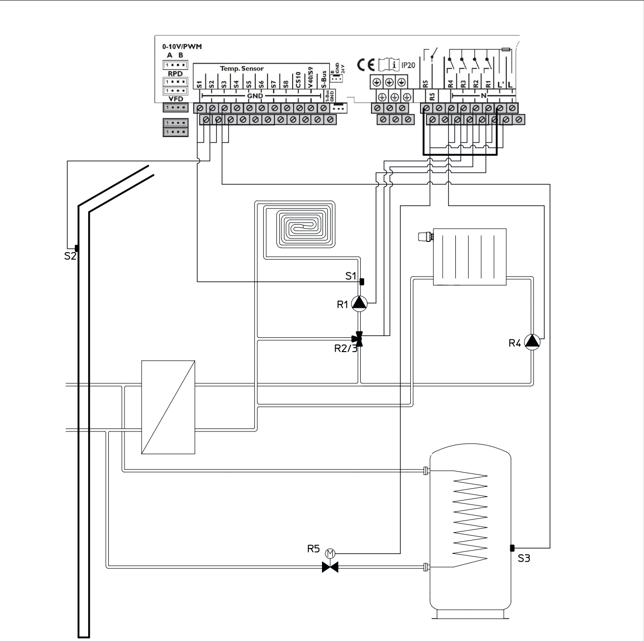
Fig. 50: Schéma 6, un circuit de chauffage mélangé et un circuit de chauffage direct, préparation d'E.C.S. directe
