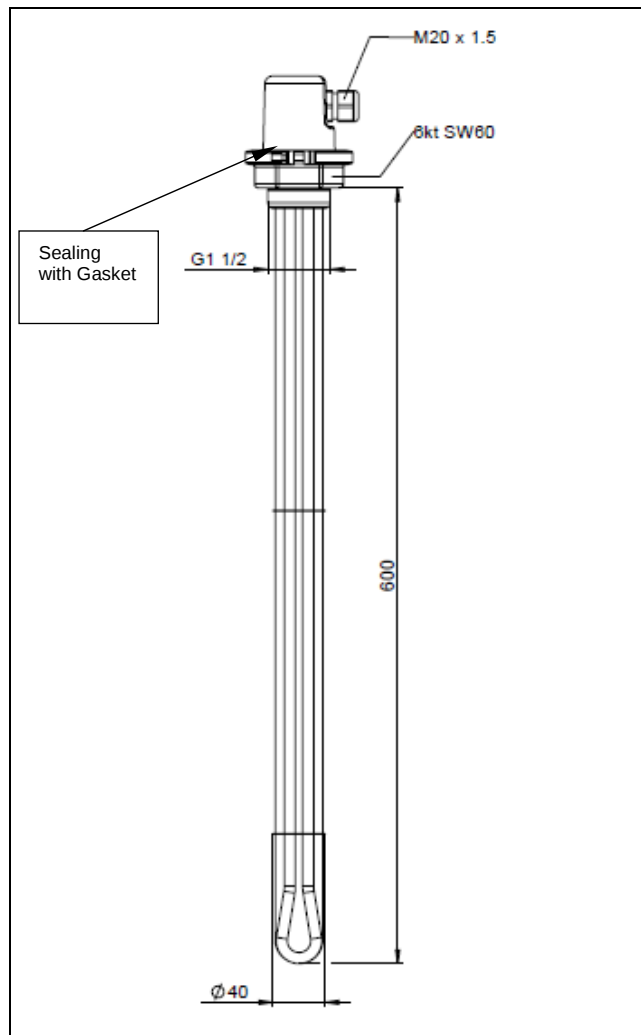
Fig. 4.1 Dimensions
