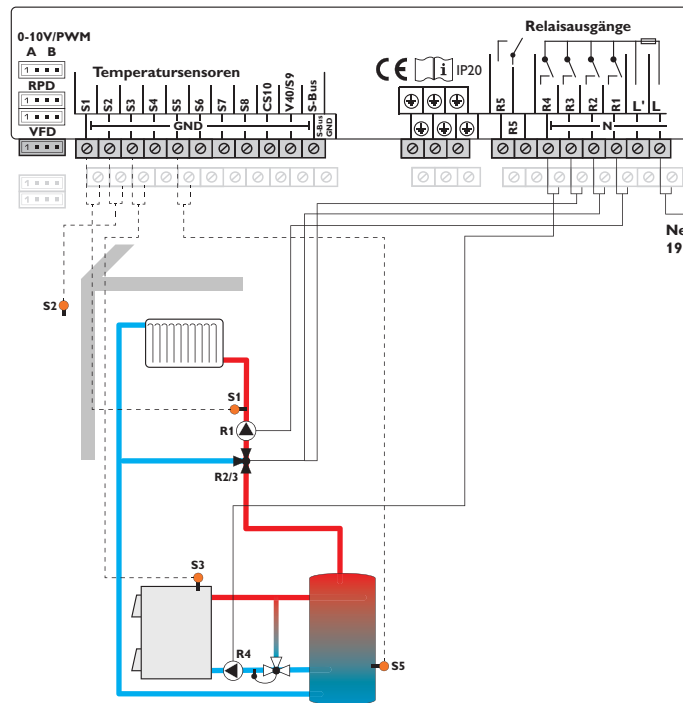
Schema 8: ein gemischter Heizkreis mit Festbrennstoffkessel
