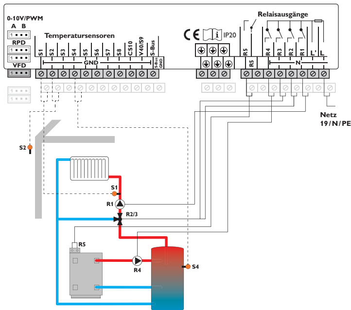
Schema 3: ein gemischter Heizkreis mit Nachheizung (Anforderung und Kessel-Ladepumpe)
