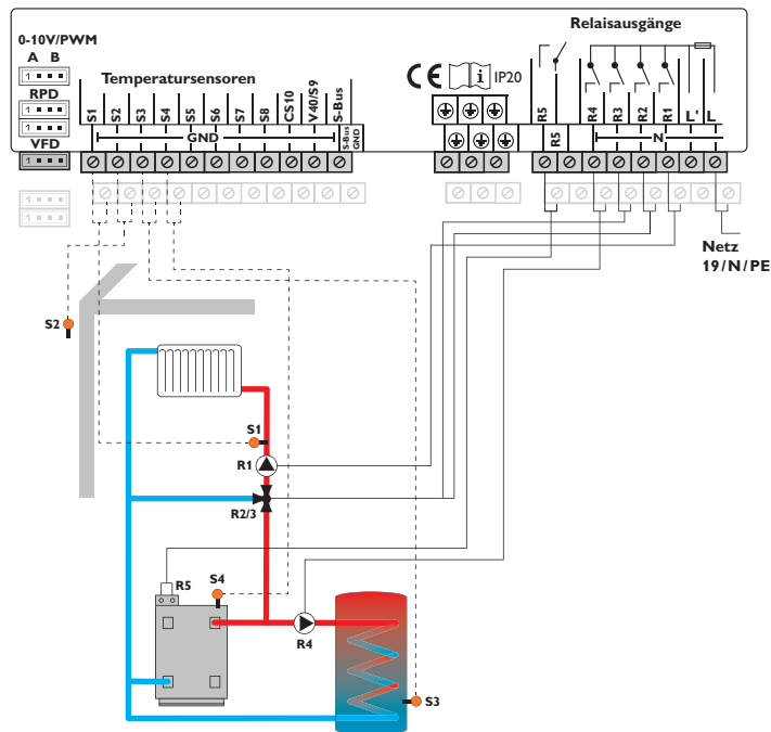
Schema 5: ein gemischter Heizkreis mit Brauchwassererwärmung und Nachheizung (Anforderung für Heizkreis und Brauchwasser)
