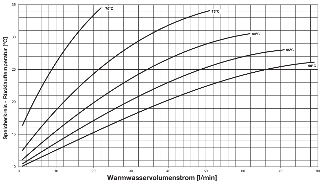
Rücklauftemperatur Speicherkreis bei unterschiedlichen Vorlauftemperaturen - Trinkwassererwärmung von 10 °C auf 70 °C -
