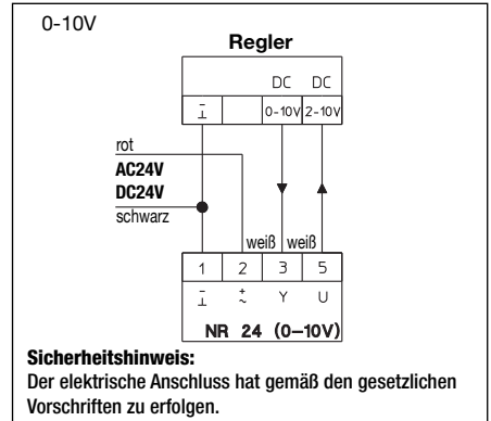
Anschluss-Schema
