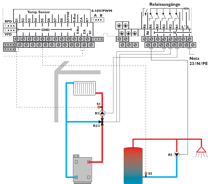
Schema 11: ein gemischter Heizkreis mit zentralem Außentemperatursensor und Zirkulation (Slave 2 ... 20)
