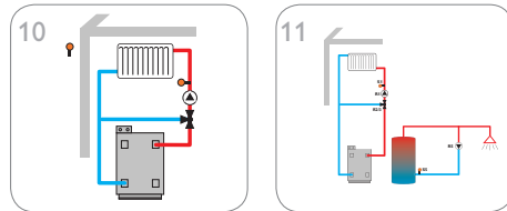
Ein gemischter Heizkreis mit zentralem Außensensor (Slave)
