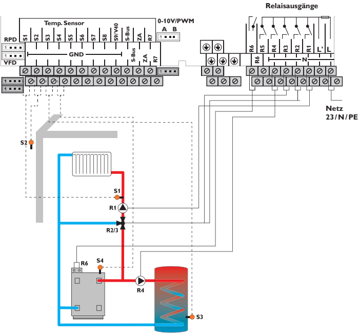
de Schema 5: ein gemischter Heizkreis mit Brauchwassererwärmung und Nachheizung (Anforderung für Heizkreis und Brauchwasser)
