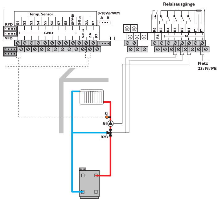
Schema 10: ein gemischter Heizkreis mit zentralem Außentemperatursensor (Slave 2...20)
