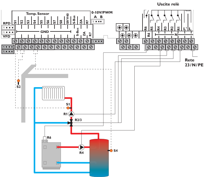
Schema 3: un circuito di riscaldamento miscelato con riscaldamento integrativo (richiesta e pompa di carico della caldaia)
