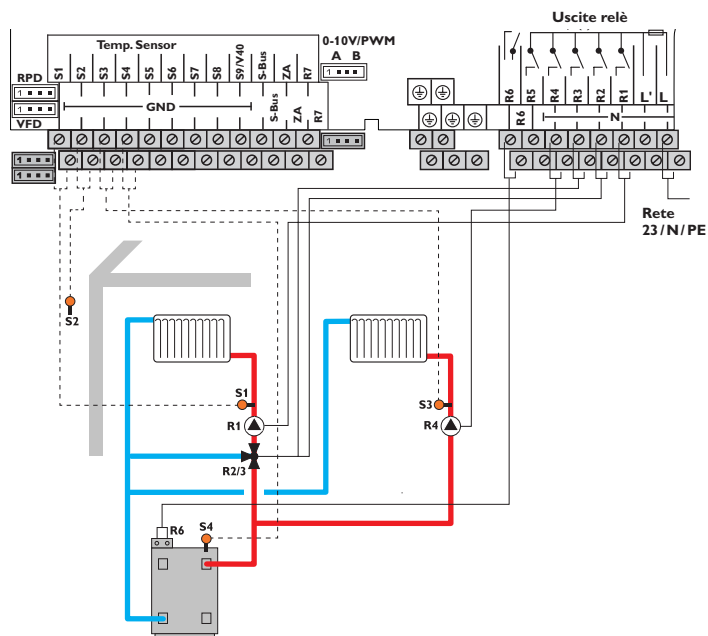
Schema 7: un circuito di riscaldamento miscelato e un circuito di riscaldamento non miscelato con riscaldamento integrativo (richiesta)
