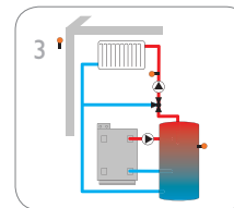
Un circuito di riscaldamento miscelato con riscaldamento integrativo e pompa di carico
