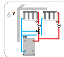
Un circuito di riscaldamento miscelato e un circuito di riscaldamento non miscelato
