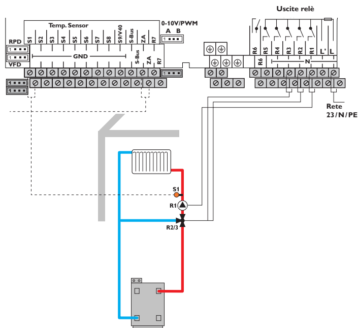
Schema 10: un circuito di riscaldamento miscelato con sensore di temperatura esterna centralizzato (slave 2... 20)
