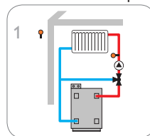
Un circuito di riscaldamento miscelato
