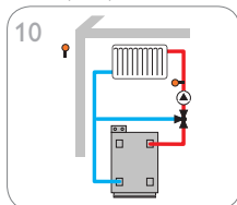
Un circuito di riscaldamento miscelato con sensore esterno centralizzato (slave)
