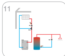
Un circuito di riscaldamento miscelato con sensore esterno centralizzato (slave) e circolazione
