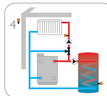
Un circuito di riscaldamento miscelato con produzione di ACS
