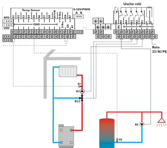
Schema 11: un circuito di riscaldamento miscelato con sensore di temperatura esterna centralizzato e circolazione (slave 2... 20)
