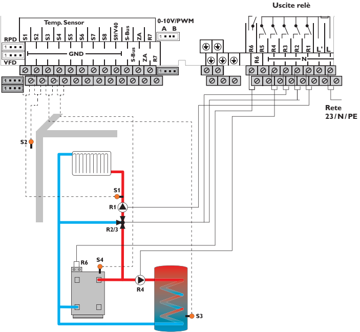
Schema 5: un circuito di riscaldamento miscelato con produzione di ACS e riscaldamento integrativo (richiesta per il circuito di riscaldamento e l'ACS)
