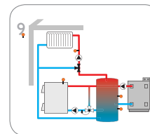
Un circuito di riscaldamento miscelato con caldaia a combustibile solido e riscaldamento integrativo
