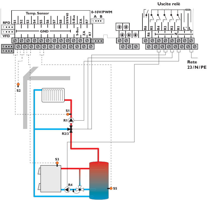
Schema 8: un circuito di riscaldamento miscelato con caldaia a combustibile solido
