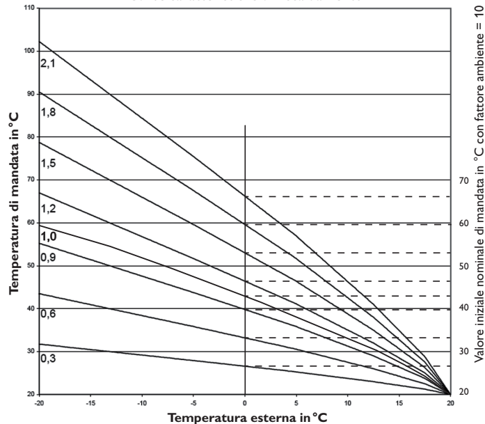
Curve caratteristiche di riscaldamento
