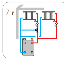
Un circuito di riscaldamento miscelato e un circuito di riscaldamento non miscelato con riscaldamento integrativo
