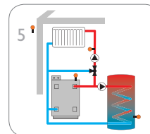
Un circuito di riscaldamento miscelato con produzione di ACS e riscaldamento integrativo
