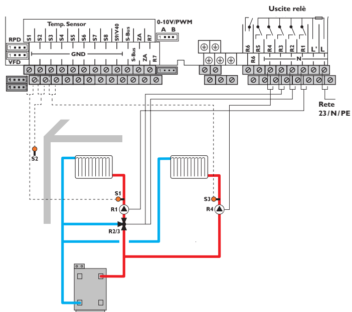
Schema 6: un circuito di riscaldamento miscelato e un circuito di riscaldamento non miscelato
