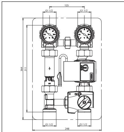
Abb. 4.2 „Regumat M3-130“ DN 25
