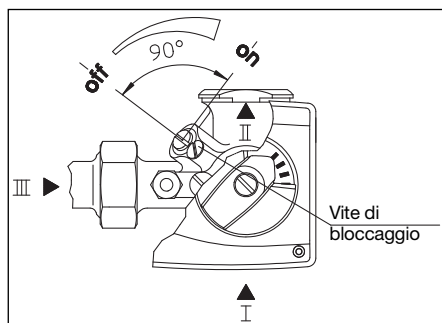
Fig. 5.2 Regolazione bypass
