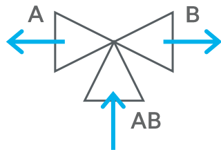
Utilisation comme robinet inverseur : Le débit AB est dévié vers A et B en fonction de la course
