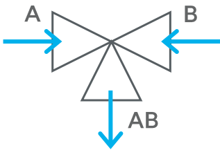
Utilisation comme robinet mitigeur : Les débits A et B sont mélangés vers AB en fonction de la course
