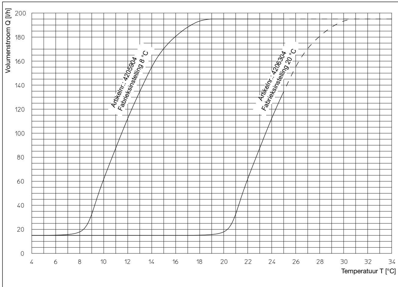
Regelkarakteristiek "Aquaström K" (gemeten bij \Delta P = 100 mbar)
