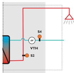
Circuito secundario
