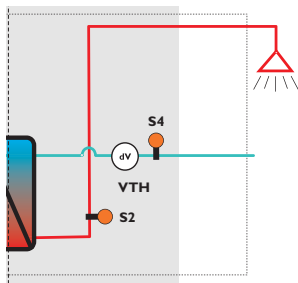
Circuito secundario
