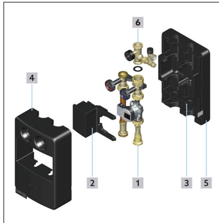
Fig. 6.6 Esplosione componenti
