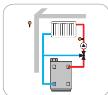
Circuit de chauffage mélangé avec sonde extérieure centrale (esclave)
