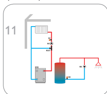
Circuit de chauffage mélangé avec sonde extérieure centrale (esclave) et circulation
